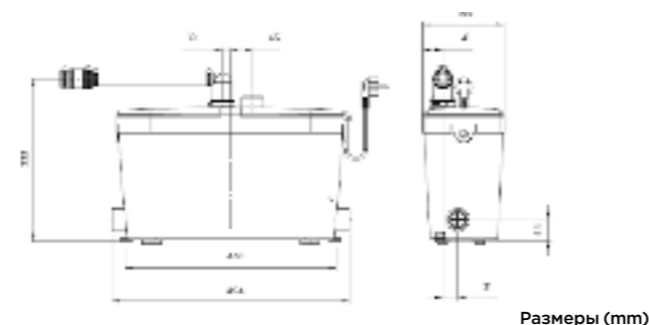
Размеры (mm)
